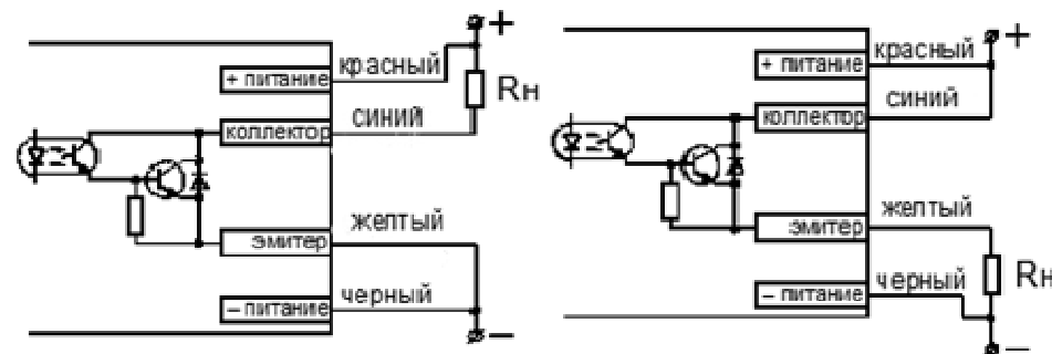
Рис.2. Схемы подключения приемника МикРА Ф15П.
