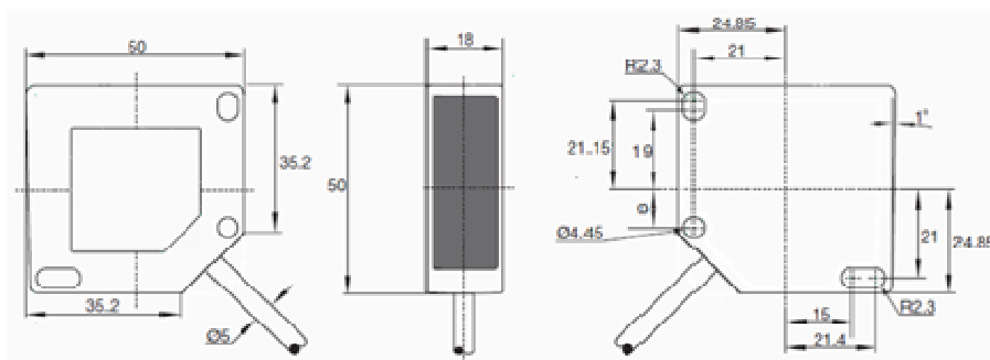
Рис.1. Габаритные размеры излучателя МикРА Ф15И и приемника МикРА Ф15П
