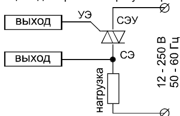
Рис.2. Схема подключения симисторов TC122-25, TC142-80.
