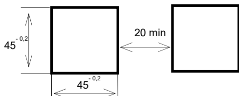
Рис.1. Вырез в щите для крепления регулятора.
