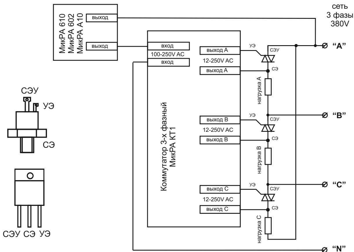
Схема подключения 3-х фазной нагрузки по схеме «Треугольник» к регуляторам температуры МикРА с использованием коммутатора МикРА КТ1 и симисторов TC16, TC122, TC132, TC142, TC171, BT139, BTA40, BTA41
