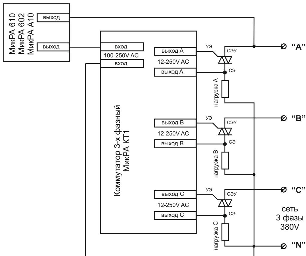
Схема подключения 3-х фазной нагрузки по схеме «Звезда» к регуляторам температуры МикРА с использованием коммутатора МикРА КТ1 и симисторов TC16, TC122, TC132, TC142, TC171, BT139, BTA40, BTA41
