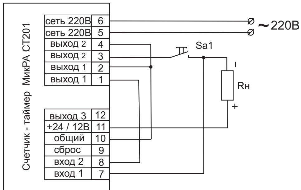
Питание нагрузки от встроенного источника напряжения +24В (+12В) током до 100мА
