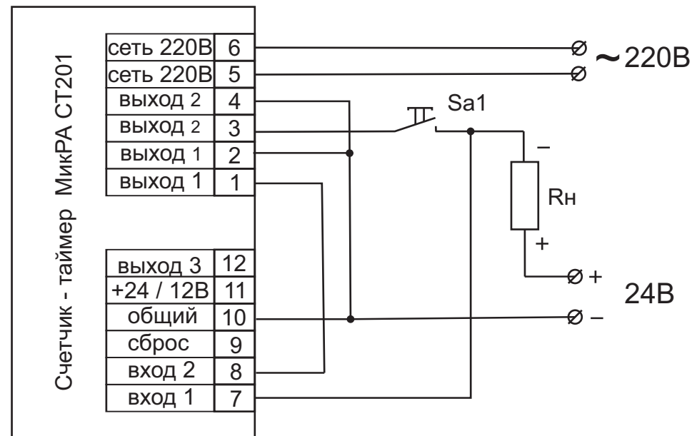
Питание нагрузки от внешнего источника постоянного напряжения от 12В до 30В
